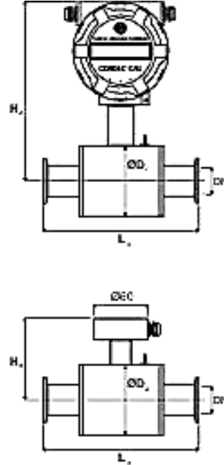
CLAMP/ FILETTO ALIM. (DIN32676/DIN11851)
