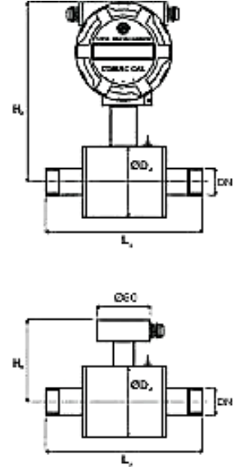
FILETTATO (EN 10226-1)
