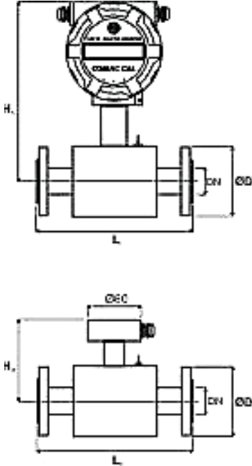
FLANGIATO (EN 1092)
